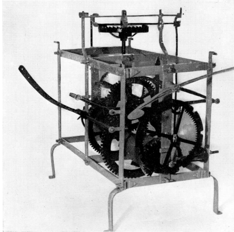
Horloge : mécanisme de la sonnerie
