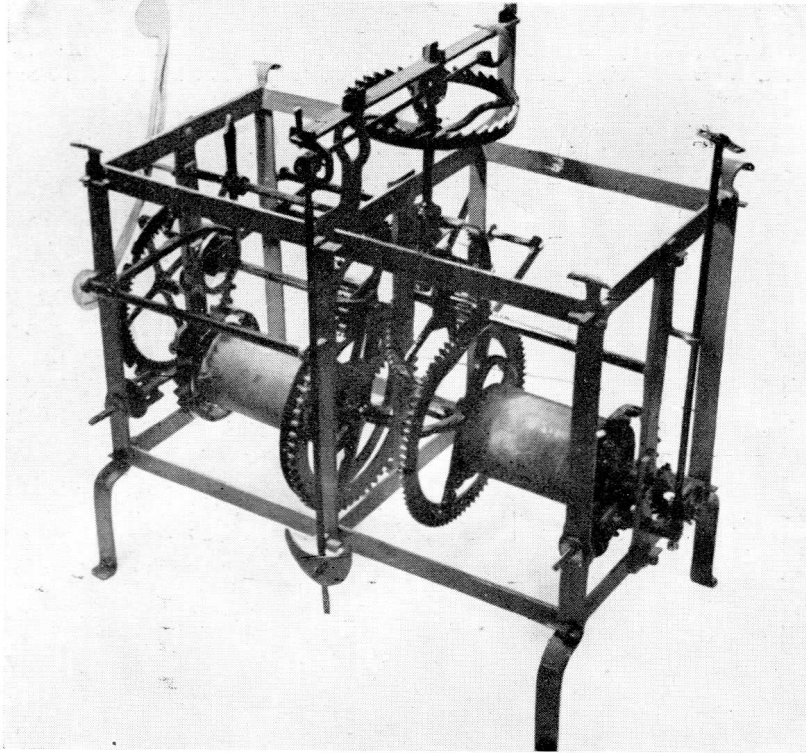
Horloge : mécanisme du mouvement
